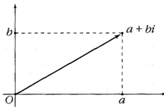
Рис. 1. Векторная форма представления комплексной величины
